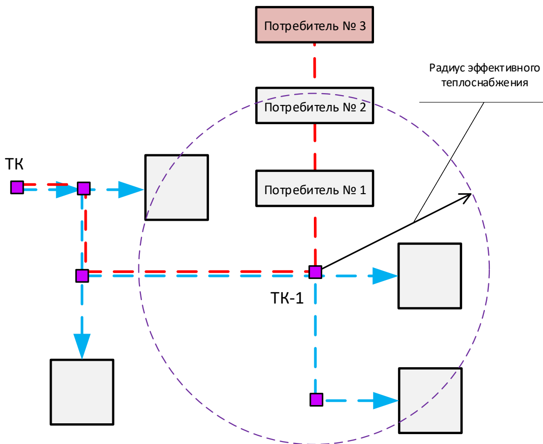
Рисунок 2 - Расчетная модель системы теплоснабжения (потребители № 1 и № 2 находятся в зоне эффективного теплоснабжения)
