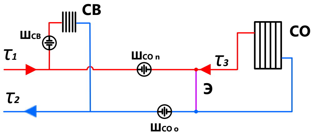
Рисунок 3 – Схема подключения потребителей к двухтрубной тепловой сети (при наличии внутридомовой системы отопления), в качестве регулятора температуры используется элеватор (СО – система отопление, Э – элеватор, СВ – система вентиляции)
