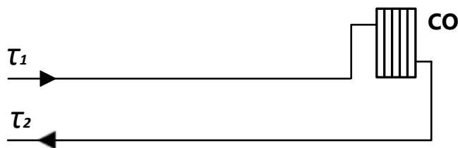
Рисунок 2 - Схема подключения потребителей к двухтрубной тепловой сети (при наличии внутридомовой системы отопления), зависимое присоединение, без смешения
