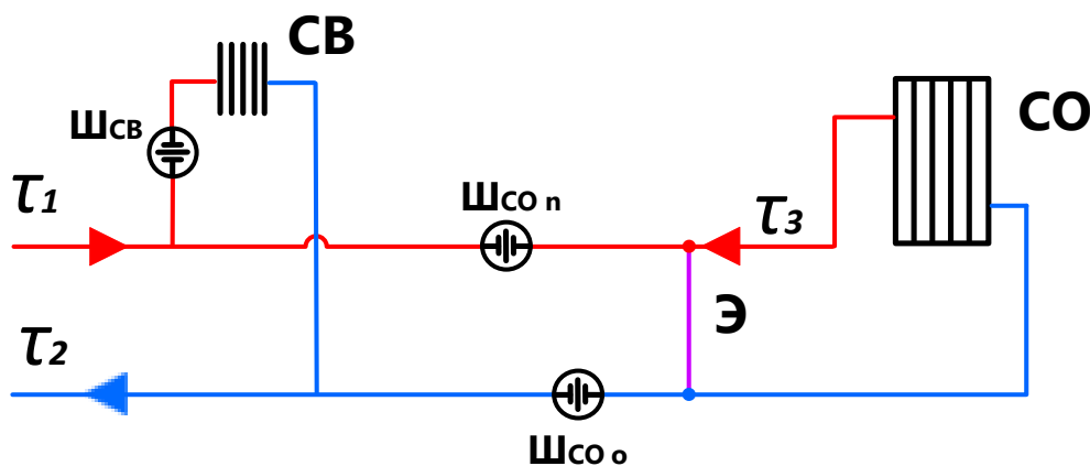
Рисунок 3 – Схема подключения потребителей к двухтрубной тепловой сети (при наличии внутридомовой системы отопления), в качестве регулятора температуры используется элеватор (СО – система отопления, Э – элеватор, СВ – система вентиляции)
